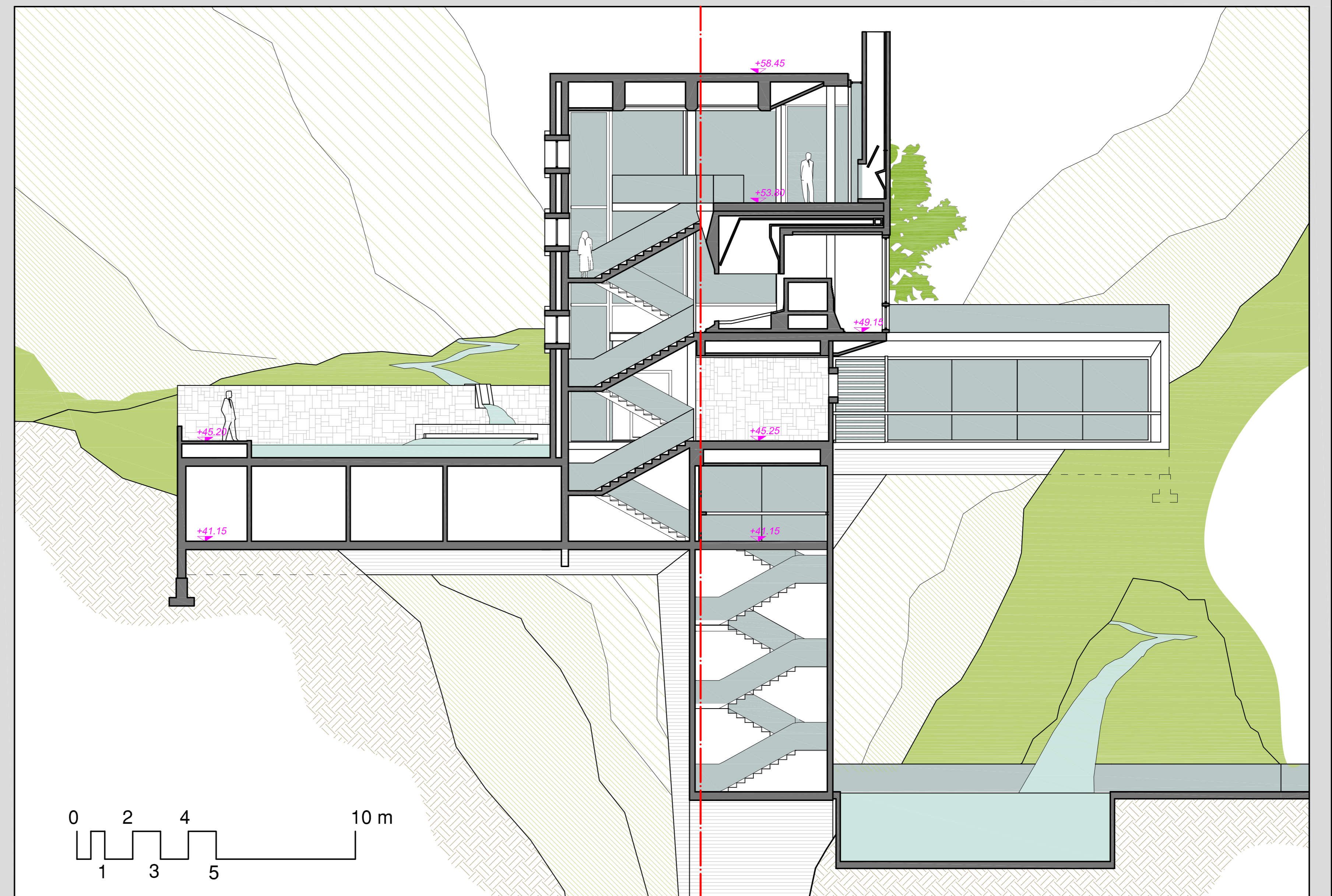
sezione AA
