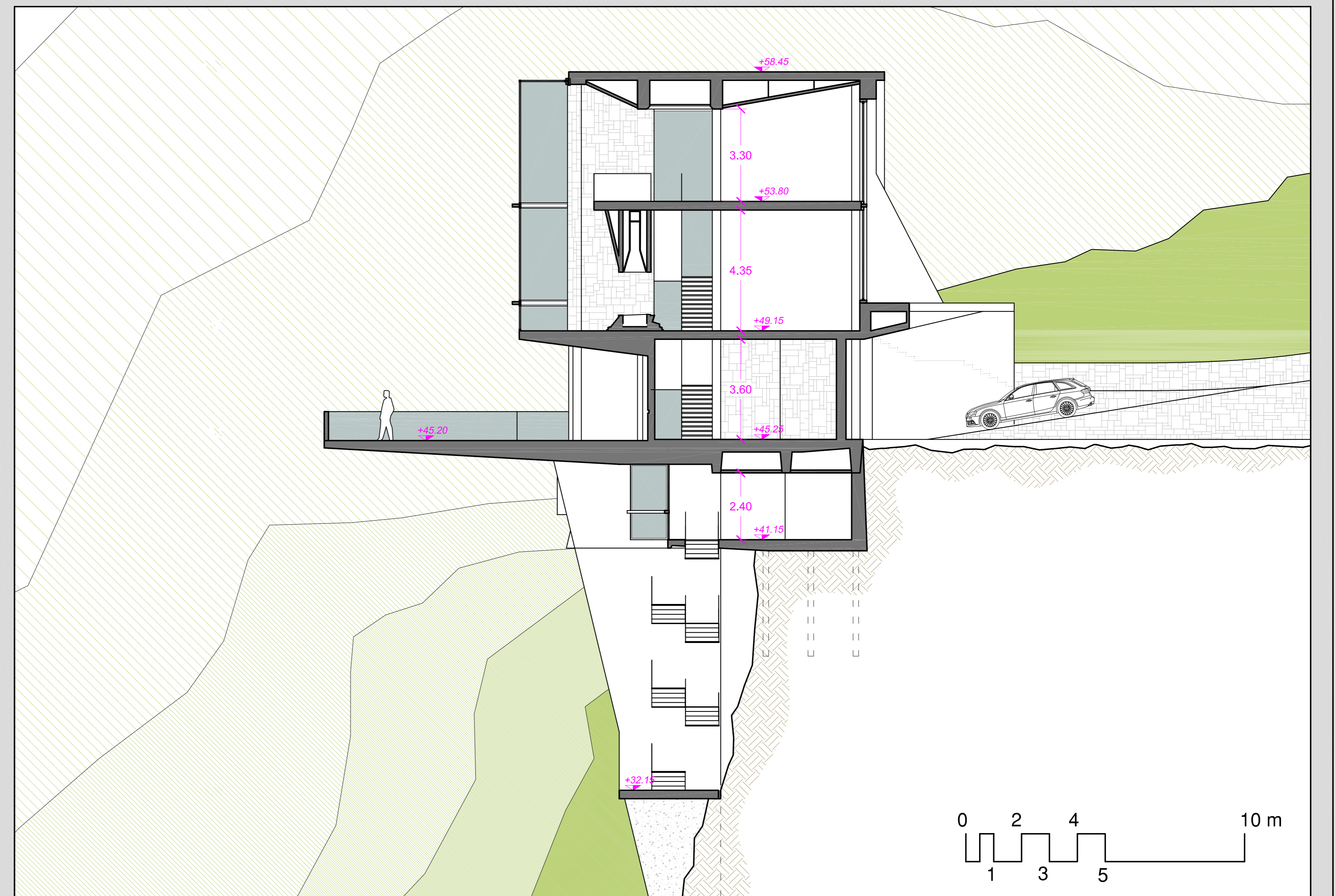
sezione CC
