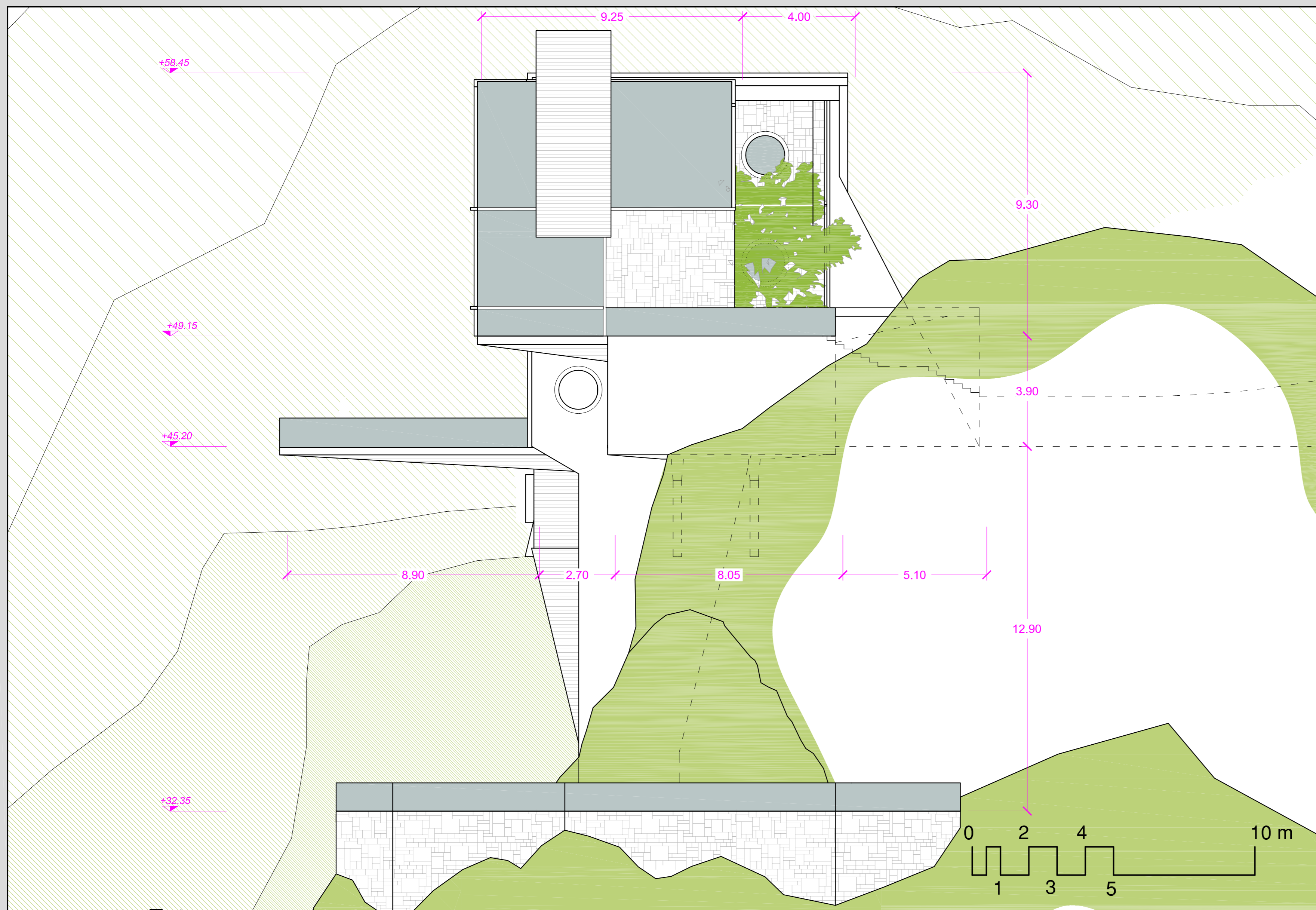
prospetto Est
