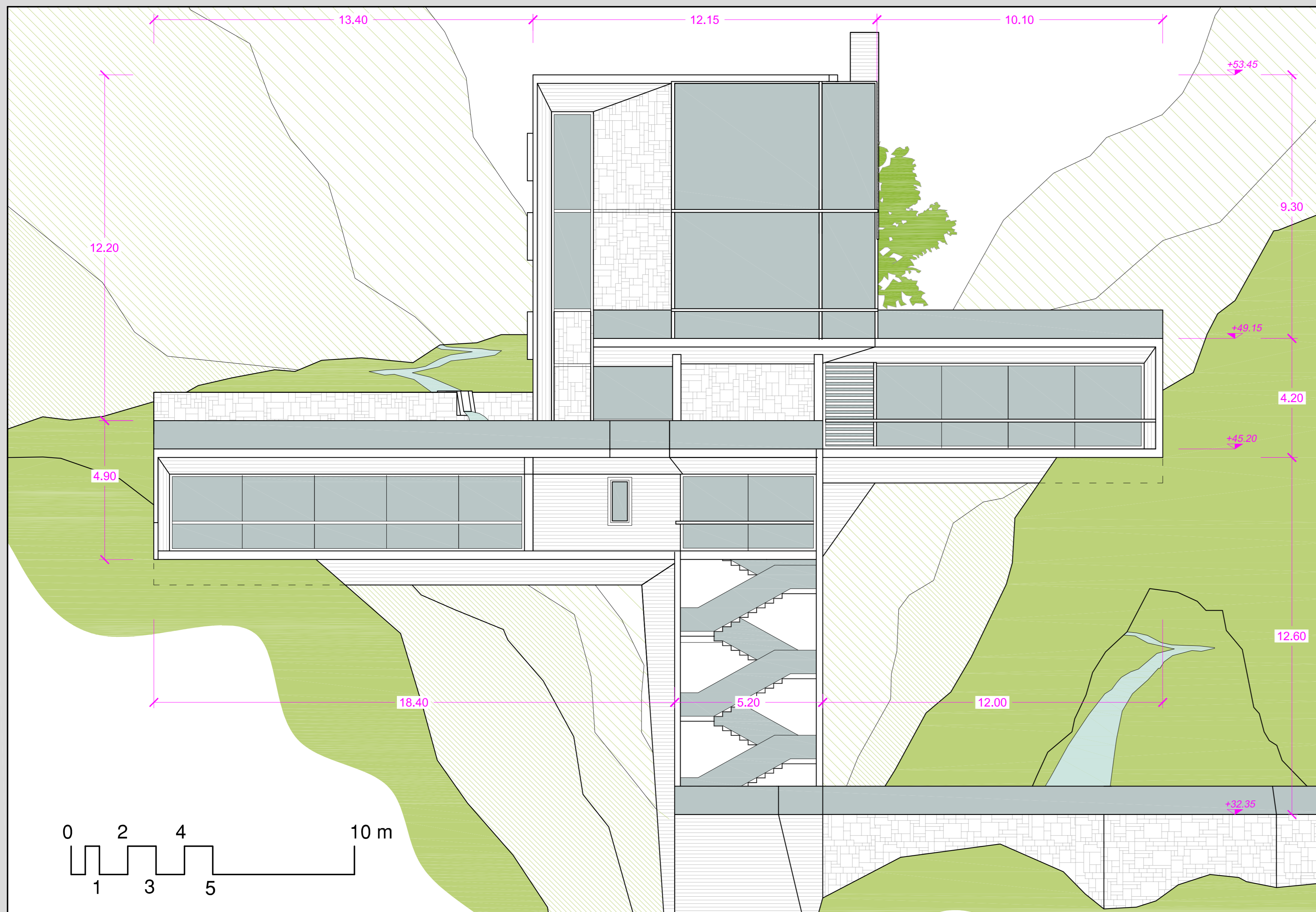
prospetto Sud
