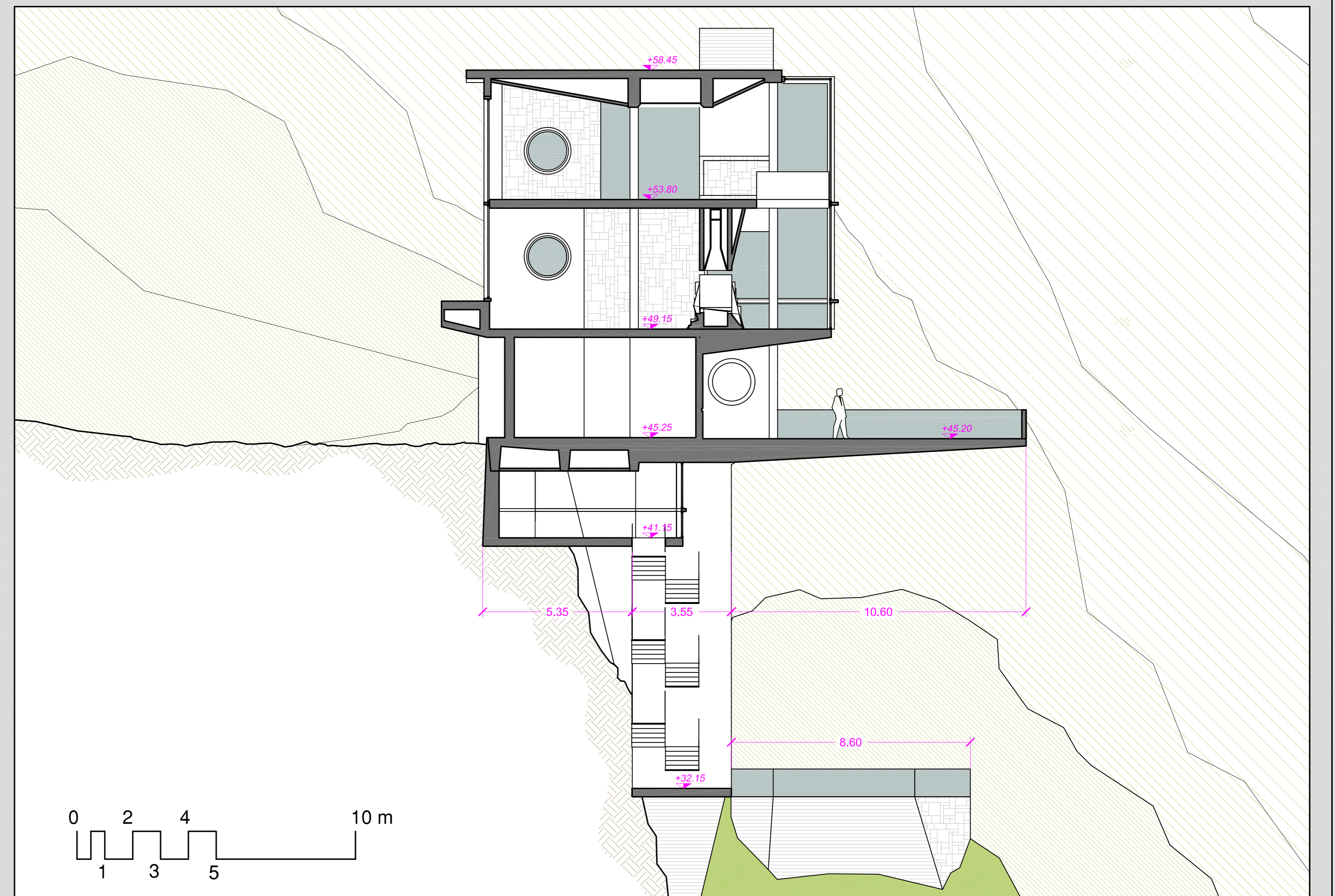
sezione BB
