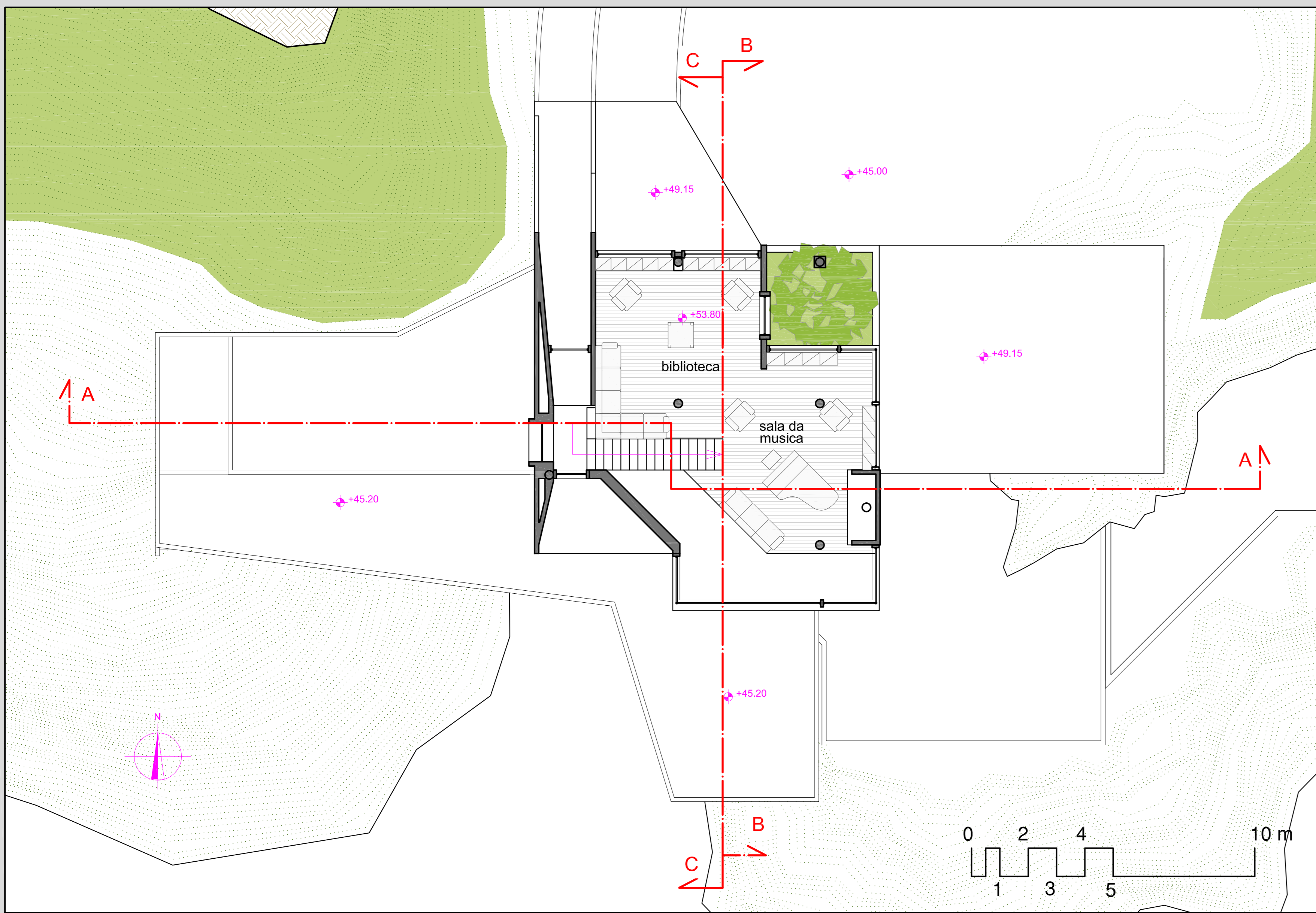
livello 03
