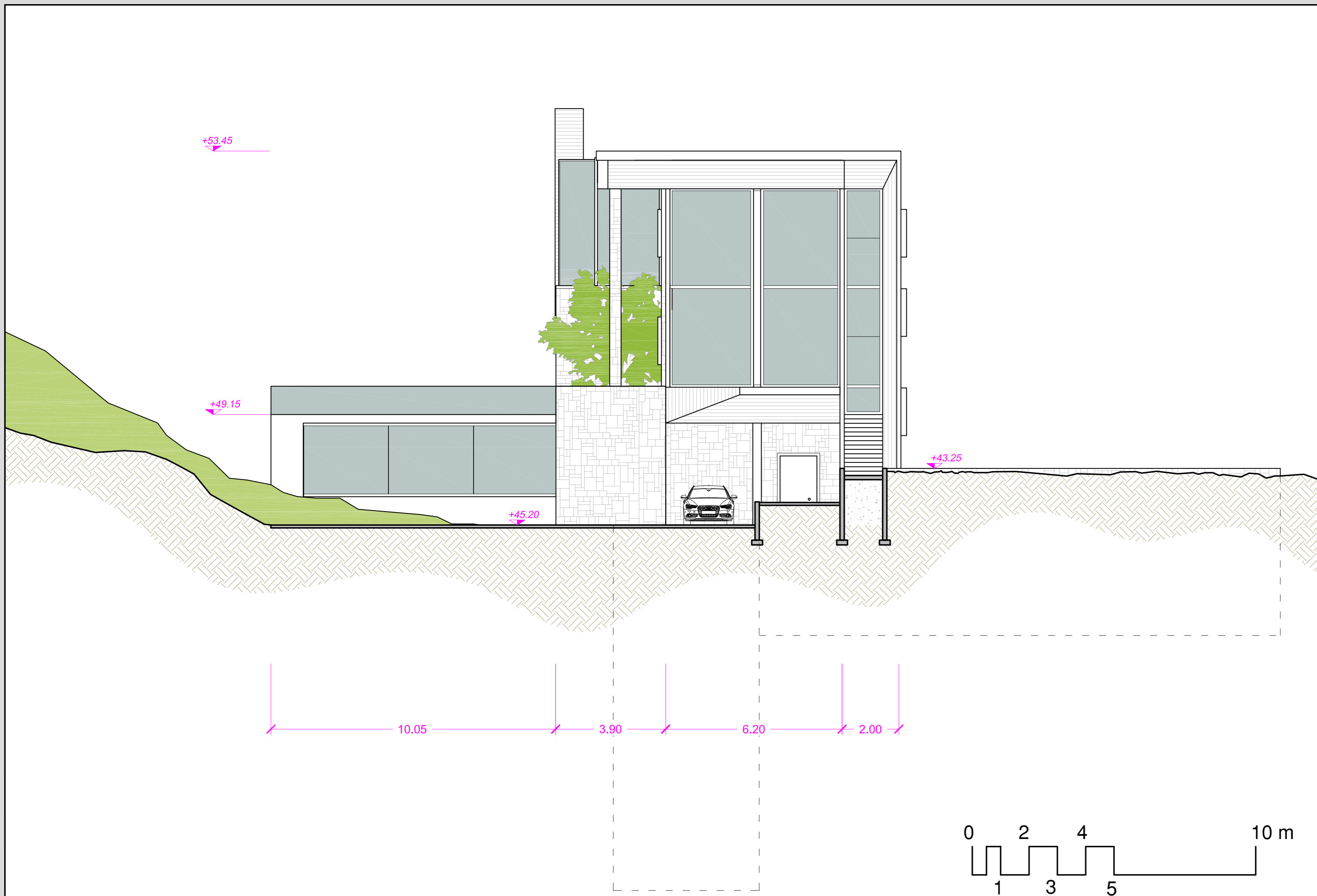
prospetto Nord
