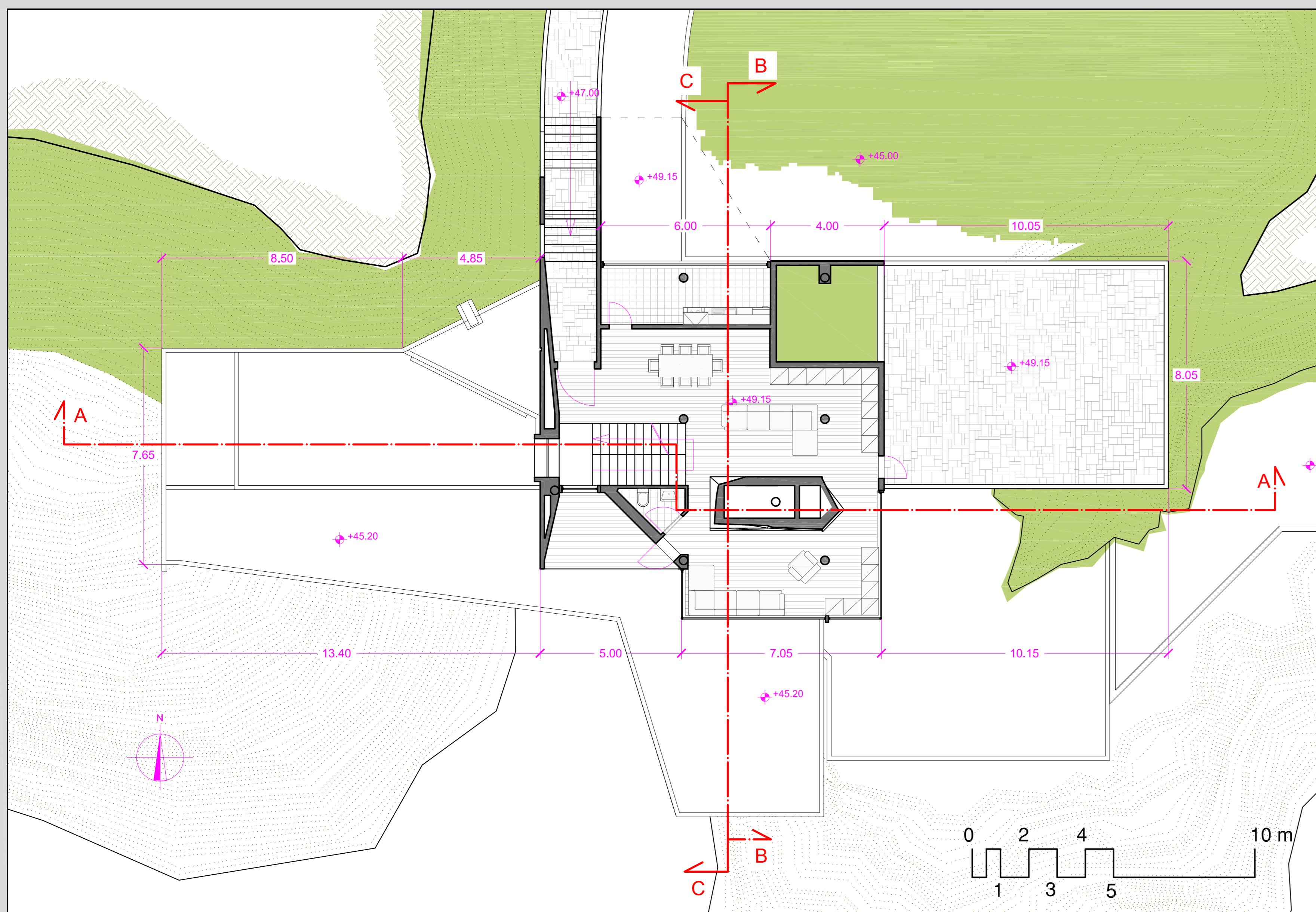
livello 02
