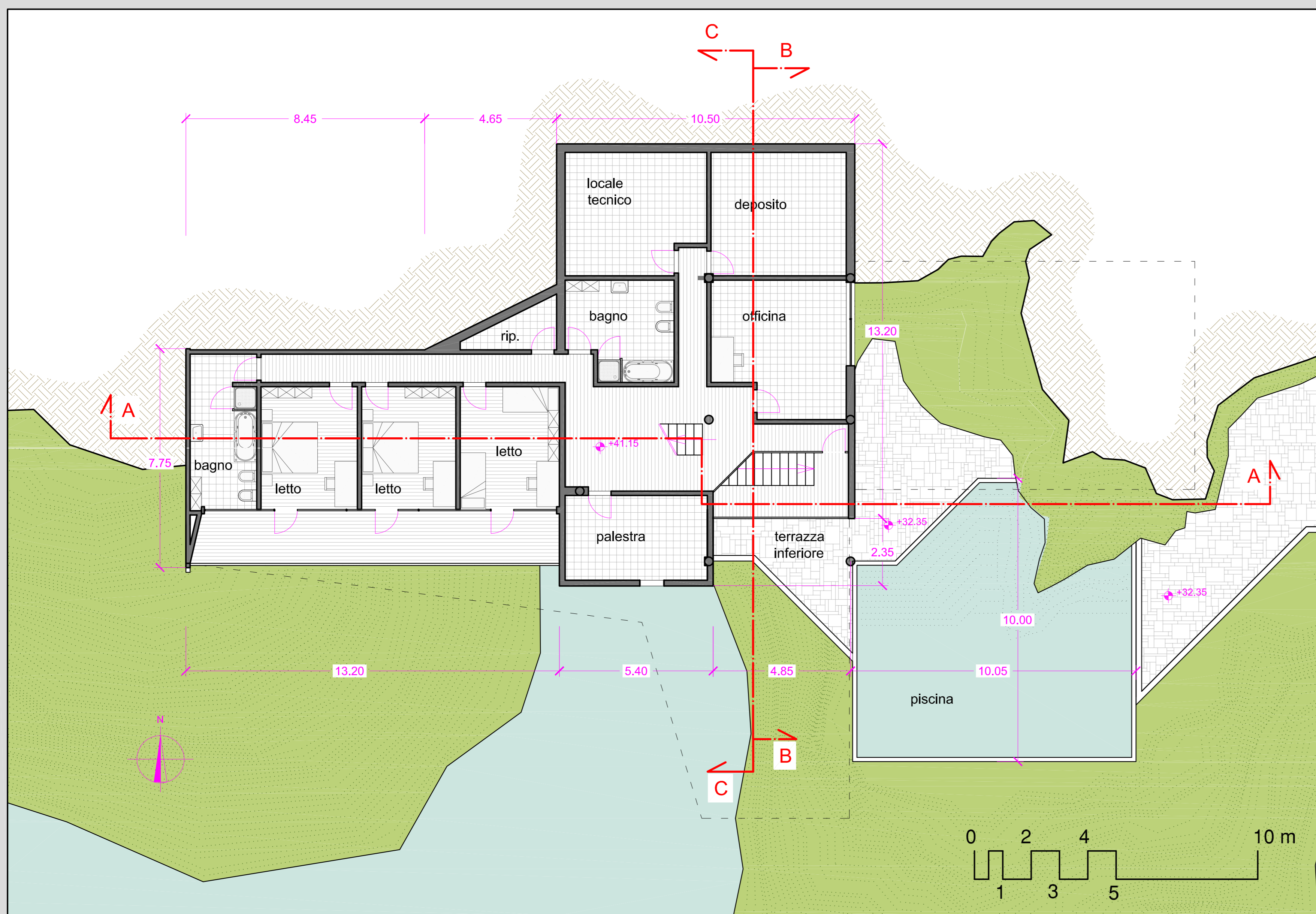
livello 0
