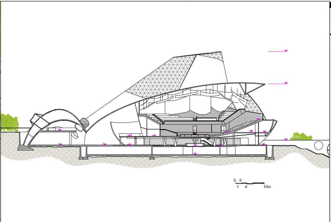
sezione CC
