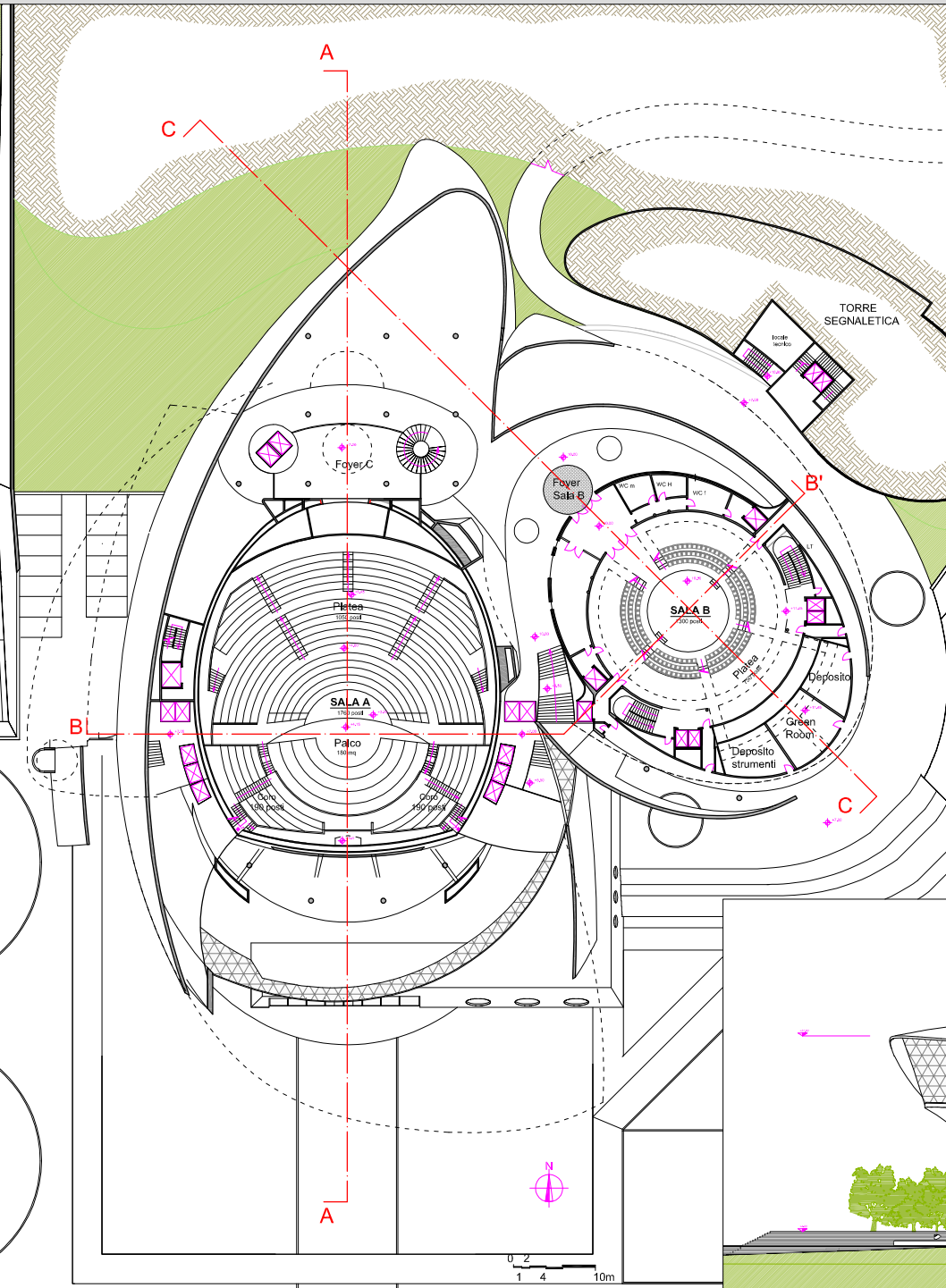
livello +10.00M
