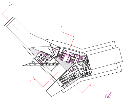
Piani 48 - 52 Uffici
