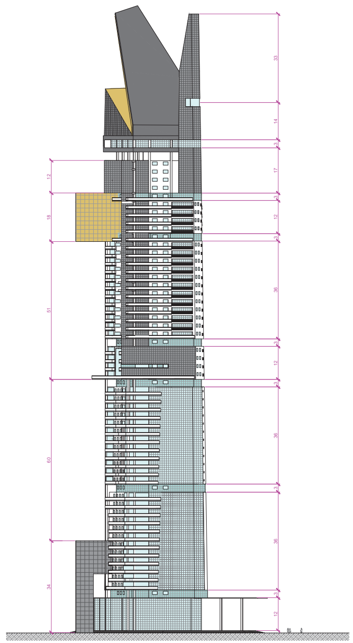
Prospetto Est 1:500
