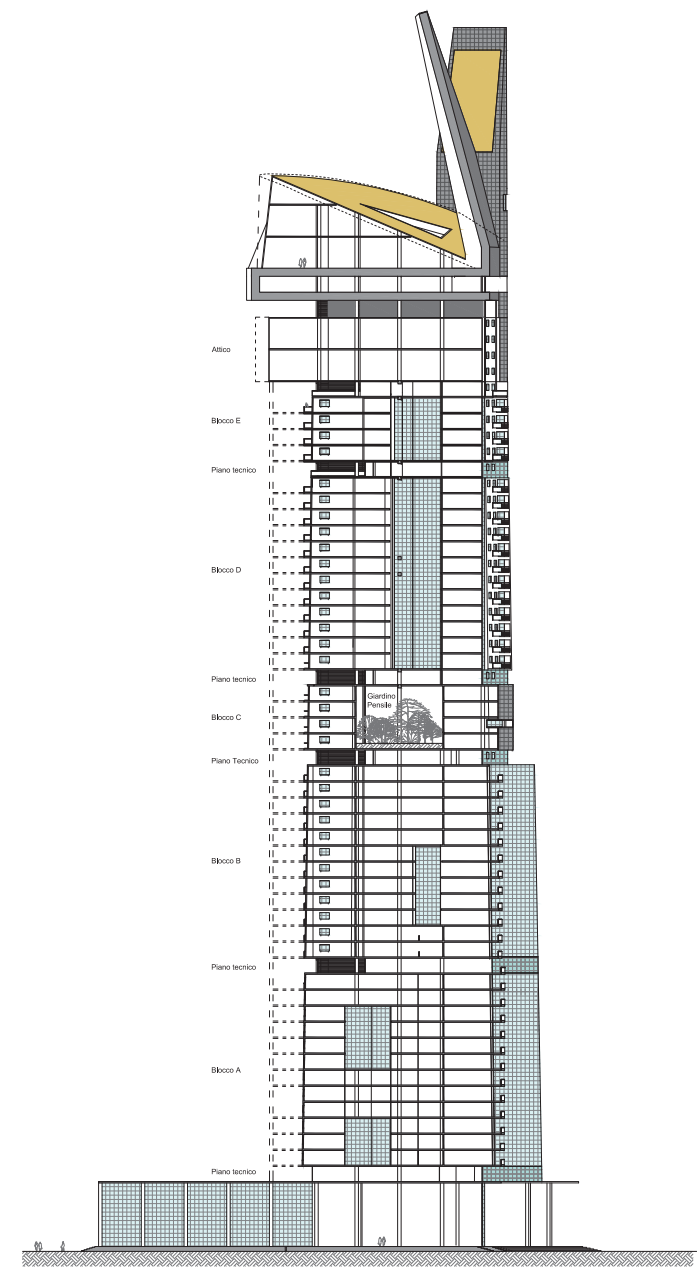
Sezione AA 1:500
