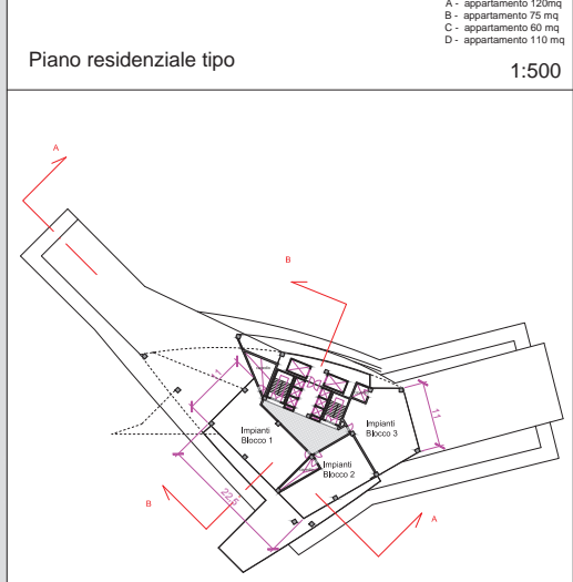
Piano Tecnico 1:500
