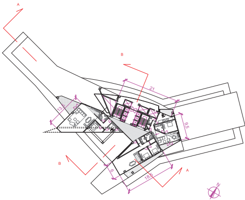
Piani 48 - 52 Appartamenti
